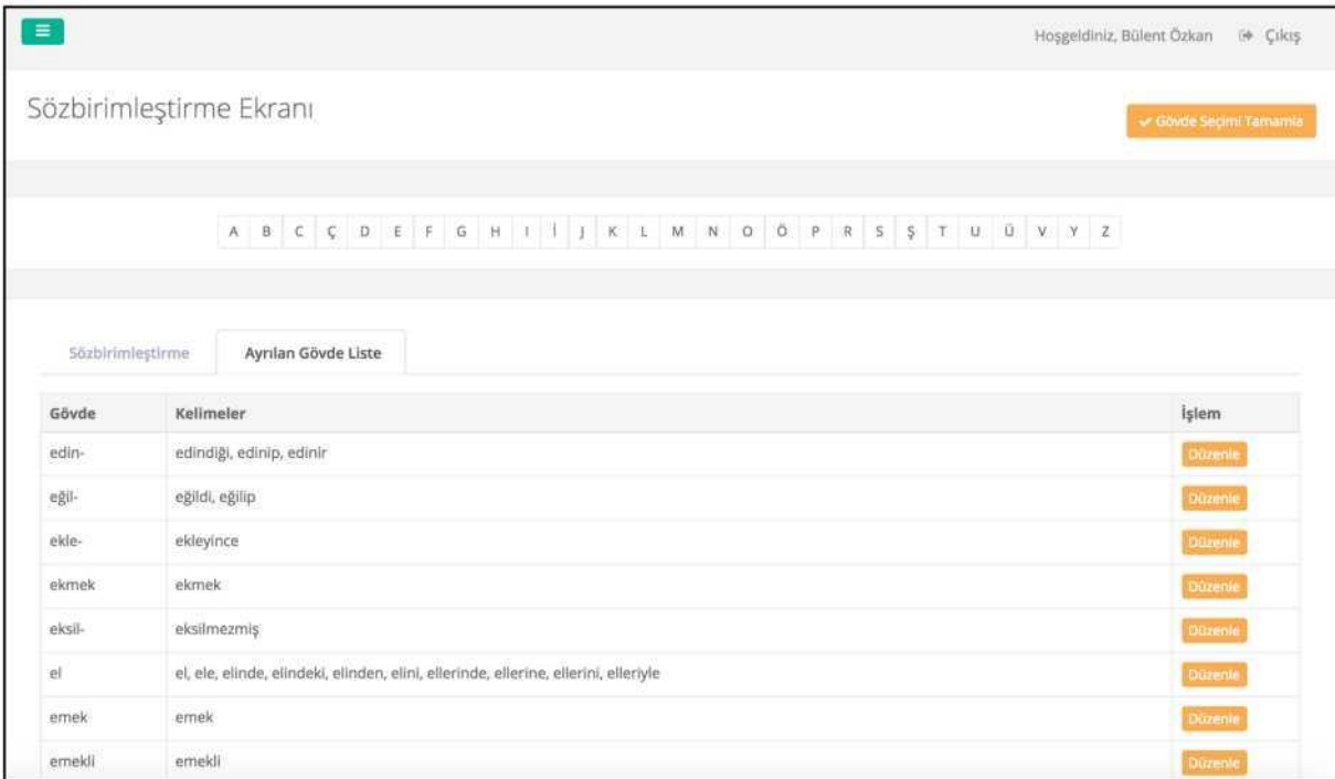
Şekil 34. Sözlük Bilim Modülü sözbirimleştirilmiş yapılar arayüzü
